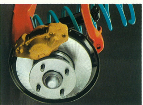
Bremskraftverstärker, Zweikreis-Bremssystem mit Scheibenbremsen vorn.
